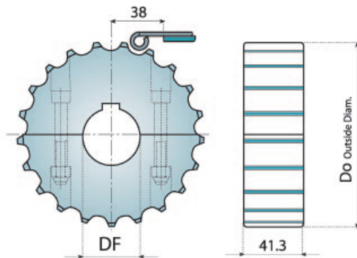
分体式主动轮 (机加工) SPLIT SPROCKETS (MACHINED)
