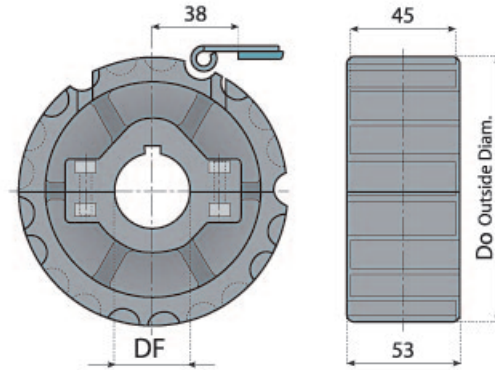
分体式主动轮 (注塑) SPLIT SPROCKETS (INJECTION)
