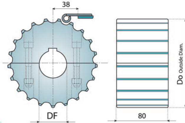
分体式主动轮 (机加工) SPLIT SPROCKETS ( MACHINED )
