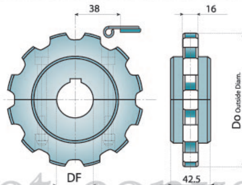
分体式主动轮 (机加工) SPLIT SPROCKETS (MACHINED)
