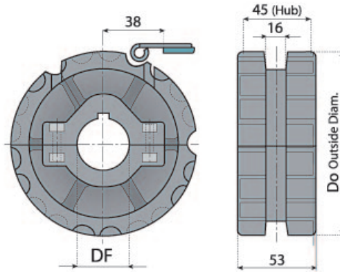
适用于 820-LBP831 链条 FOR 820-LBP831
