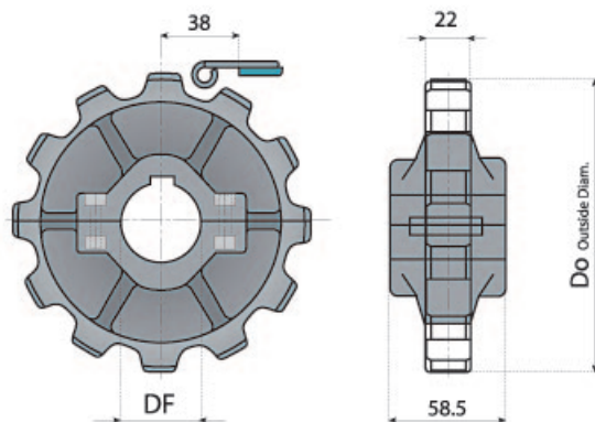
分体式从动轮 (注塑) SPLIT SPROCKETS (INJECTION)
